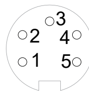
电源7/8"接口母插（金属接口）- XD2
