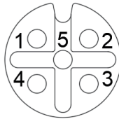
热电阻信号接口
