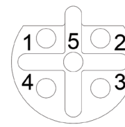
接口总线D扣母插（金属接口）- XF1/XF2
